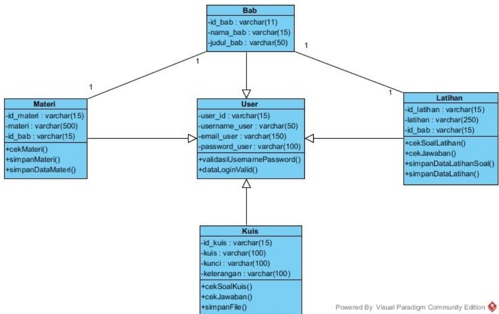
Gambar 2. Class Diagram Sistem Yang Diusulkan
